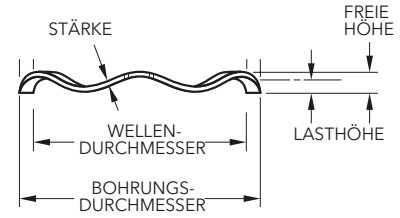
RADIALE DRAHTBREITE
